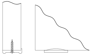
Рис.3 Схема установки эксцентриковой стяжки
