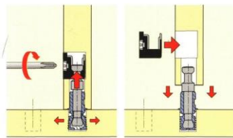
Рис.3 Схема установки эксцентриковой стяжки
