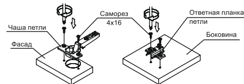
Схема 3. Установка петель
