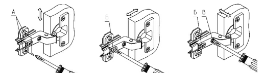
Схема 4. Регулирование положения фасада
